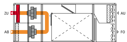
1 Umluft-Heizen-Klappe (Zusatzausrüstung)
