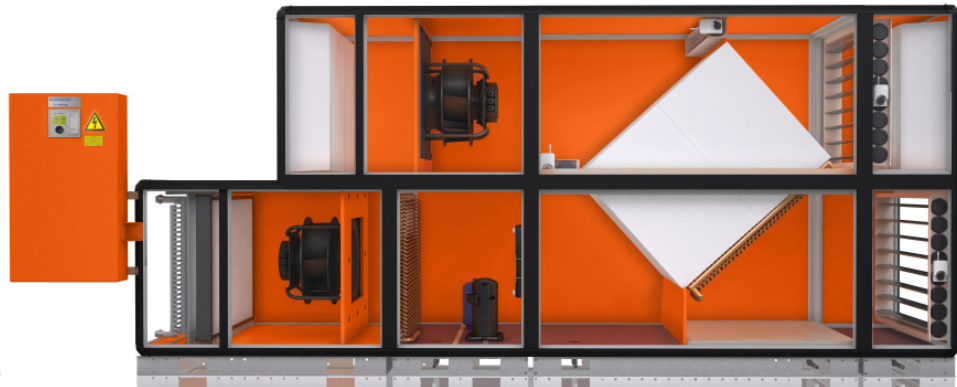
ThermoCond 39 13 01 - vereinfachte Darstellung
